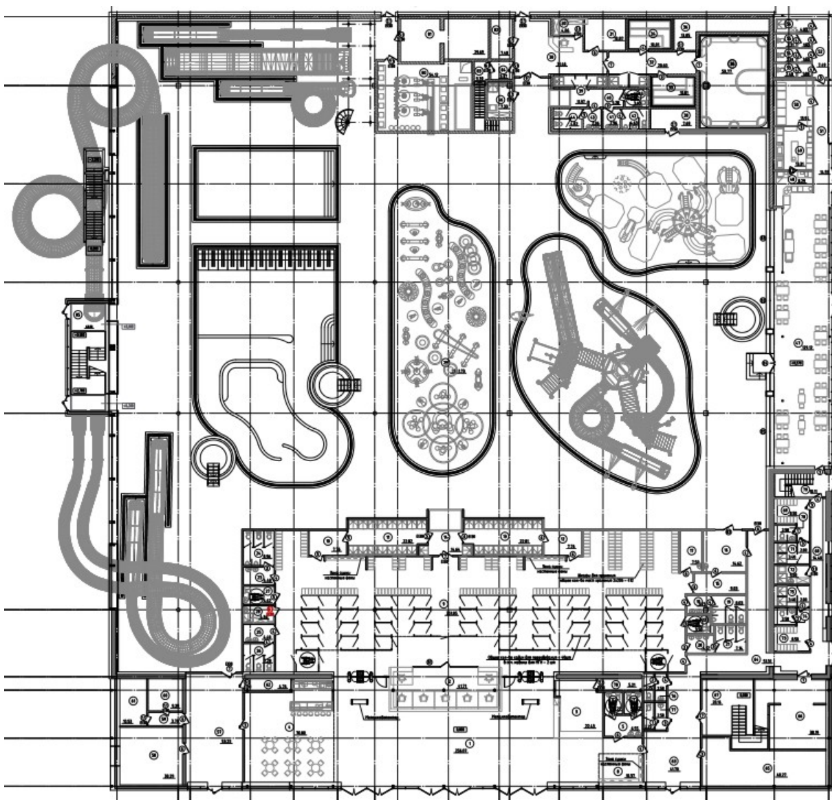
Рисунок 2 – План размещения основных объектов на территории ВПК
